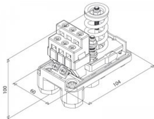
Dimensions PMA/12
